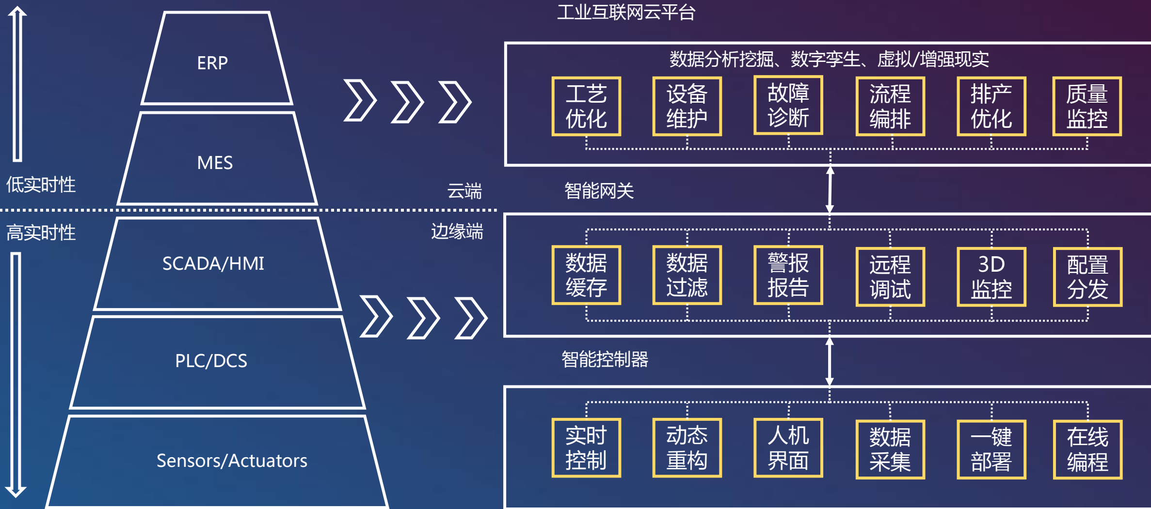
ISA-95构架
